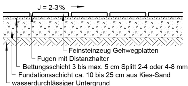
Bild 3: Aufbau des Plattenbelages über einer Foundationsschicht
