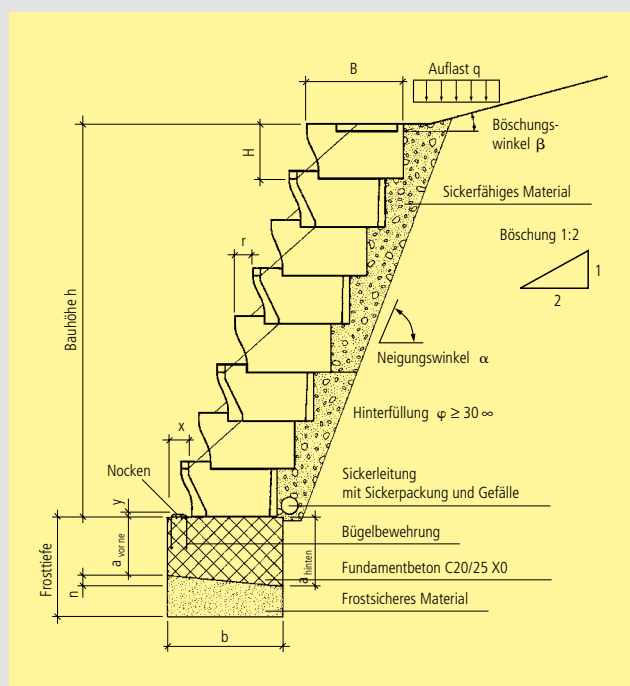
Böschungselemente Aufbau
