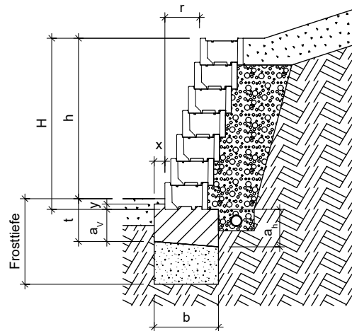
Bild 28: Lastfall D, Rücksprung 5,5 cm, \alpha = 76^\circ
