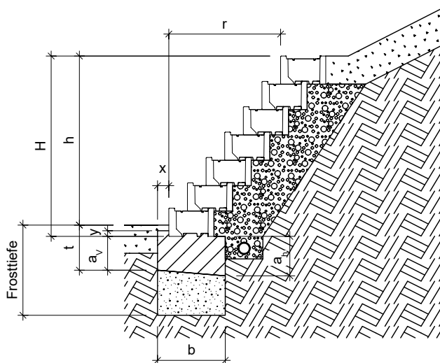
Bild 29: Lastfall E, Rücksprung 16,5 cm \alpha = 54^\circ
