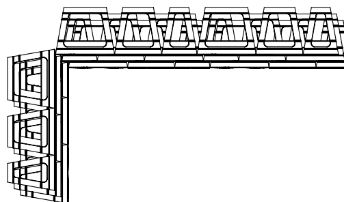
Bild 16: Grundriss Innenecke mit Rücksprung 5,5 cm
