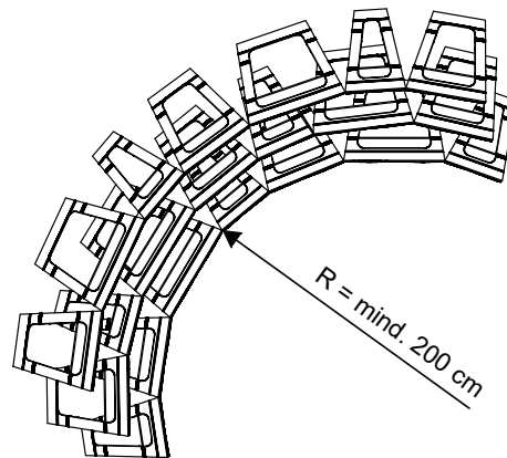
Bild 18: Grundriss Innenkurven mit Rücksprung 16,5 cm
