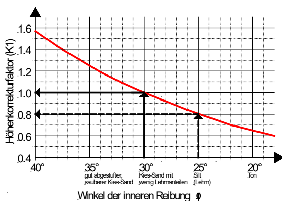
Diagramm 1: Höhenkorrekturfaktor K1
