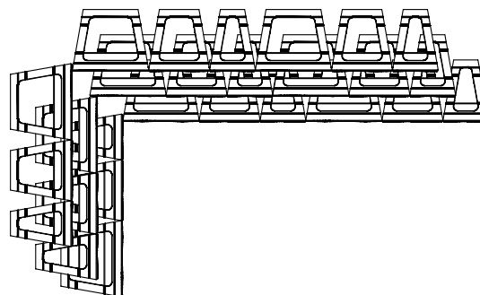
Bild 15: Grundriss Innenecke mit Rücksprung 16,5 cm
