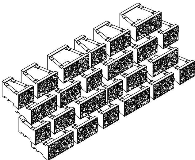
Bild 11: Isometrie Verlegemuster 3
