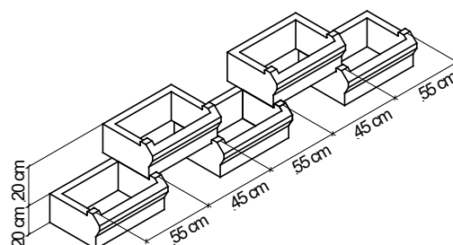
Bild 14: VERDURO® Elementabstand 45 cm (Rastermass 50 cm)
