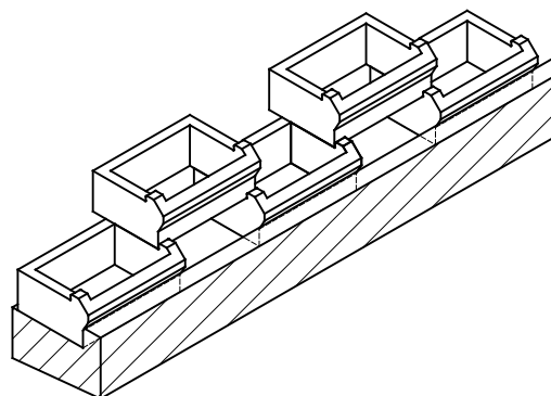
Bild 13: Fundament mit Nocken und erste Steinlage
