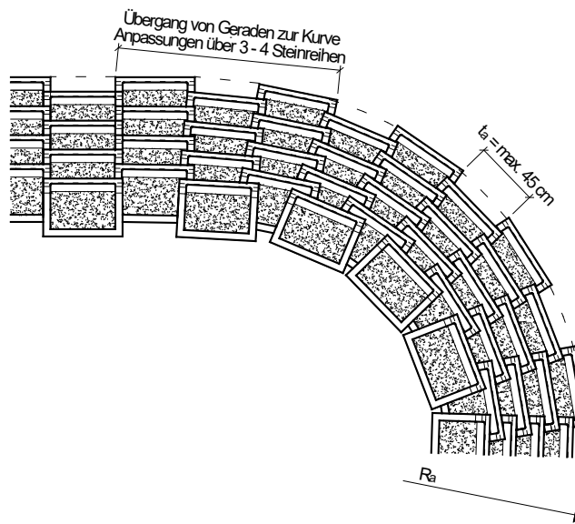
Bild 26: Aussenkurve
