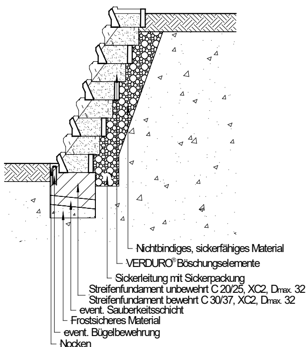
Bild 12: Aufbauquerschnitt
