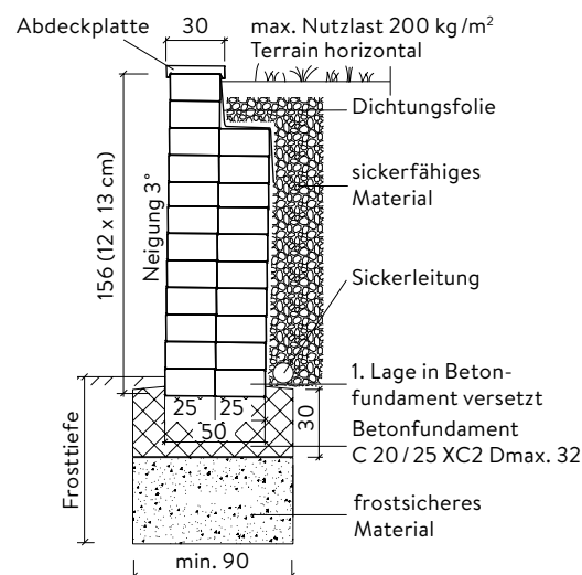
Beispiel Mauerausführung B = 50 cm ohne Geogitter
