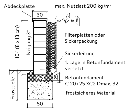
Beispiel Mauerausführung B = 25 cm ohne Geogitter
