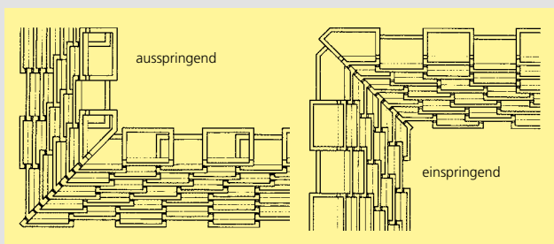
Eckenabundung
