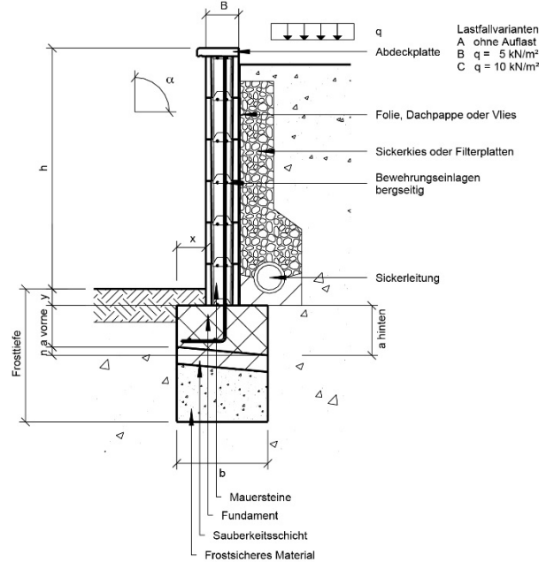
Bild 9: Aufbauquerschnitt mit Bewehrungsmöglichkeit
