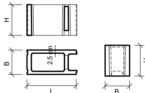
Bild 6: SCHALIT Endstein
