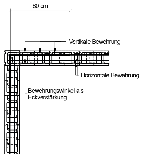
Bild 14: Eckausbildung
