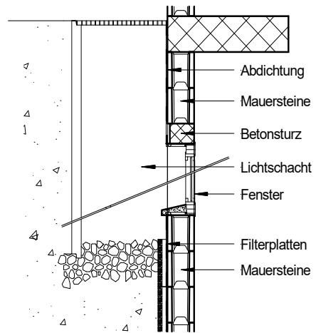
Bild 17: Querschnitt: Kellerwand mit Fenster und Betonsturz
