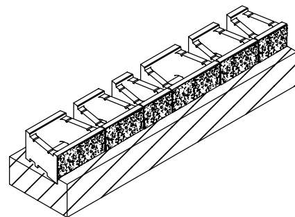
Bild 6: Fundament mit Nocken und erste Steinlage
