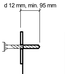
Bild 32: Loch bohren, d = 12 mm
