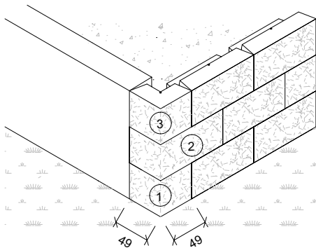
Bild 15 FELSMAUER Böschungselemente – Sichtbaren Stirnseiten links (① Anfangseckstein 1/2, ② Mitteleckstein links, ③ Schlusseckstein 1/2)
