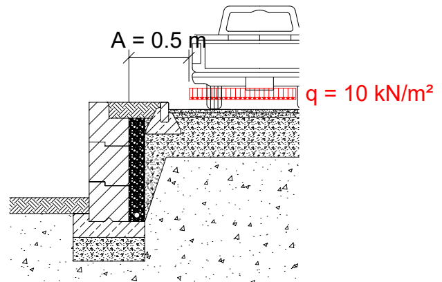
Bild 6 Lastfall C
