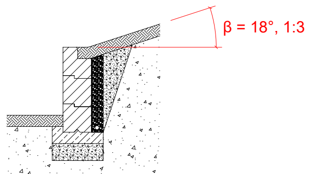
Bild 7 Lastfall D
