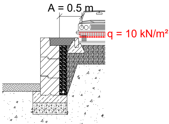
Bild 5 Lastfall B
