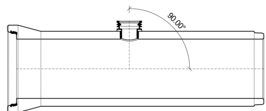
Bild 4: Anschlusswinkel DENSO Steckanschlusstück
