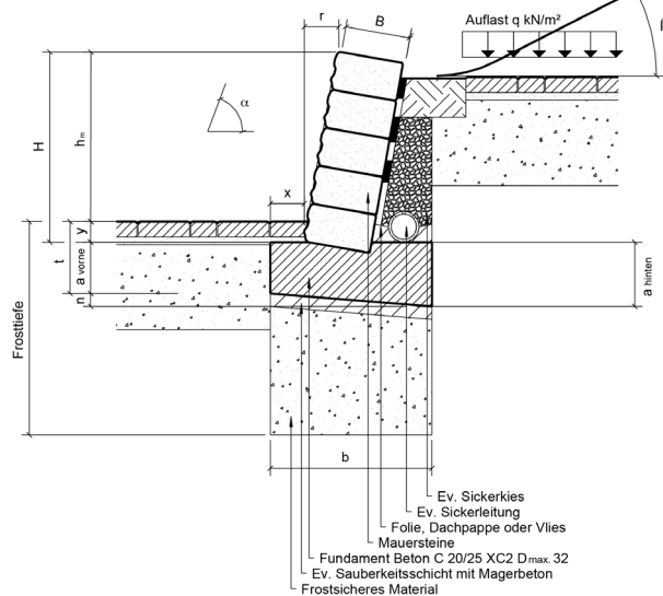
Bild 47: Geneigter Maueraufbau
