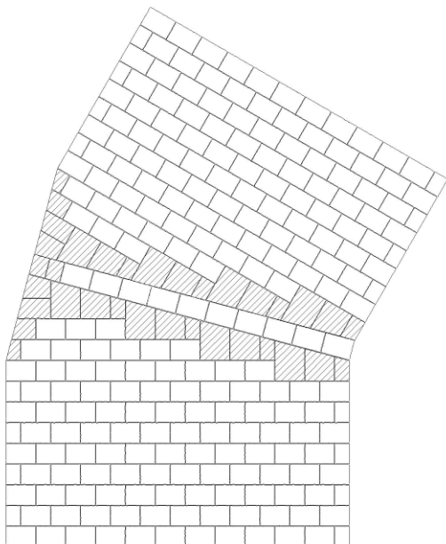
Bild 25: Mögliches Verlegebild bei Wechsel der Verlegrichtung mit TEGULA® Pflastersteinen, schraffierte Steine zeigen die zugeschnittenen Passesteine
