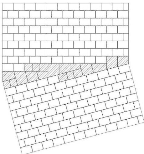
Bild 26: Mögliches Verlegebild bei Wechsel der Verlegrichtung mit TEGULA® Pflastersteinen, schraffierte Steine zeigen die zugeschnittenen Passesteine
