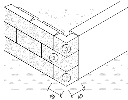
Bild 16 FELSMAUER Böschungselemente – Sichtbaren Stirnseiten rechts (① Anfangseckstein rechts, ② Mitteleckstein rechts, ③ Schlusseckstein rechts)
