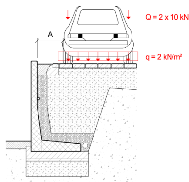
Bild 12: Lastfall B2
