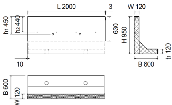
Bild 5: Perronwinkel Typ 5
