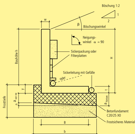
Winkelplatteneinbau
