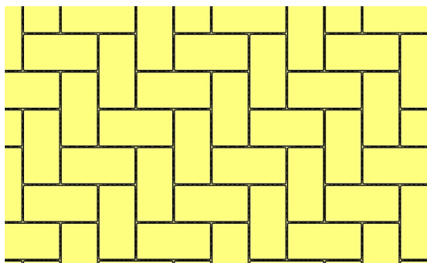
Bild 10: Geeigneter Verband bei Längsgefälle > 6% (Fischgrat)
