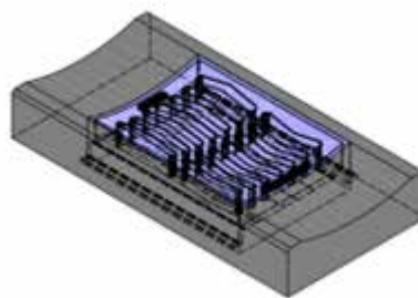
Abbildung 2 Strassenschale inkl. Gussrost C 250
