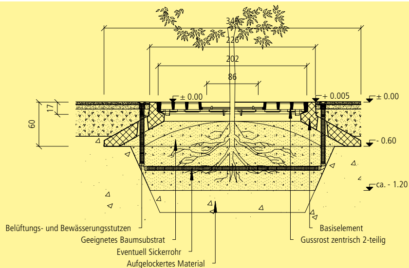
Einbauschema COPAL CUPOLA Baumwurzelraumschutz mit Gussrost
