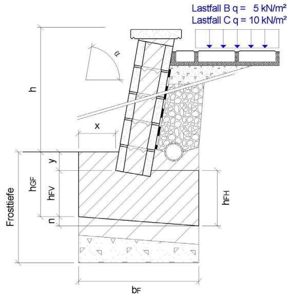
Bild 24: Schematische Darstellung einer Mauer mit horizontaler Hinterfüllung mit zusätzlicher Auflast, ohne Bewehrungseinlagen (technische Werte siehe Tabelle 15 und 17)
