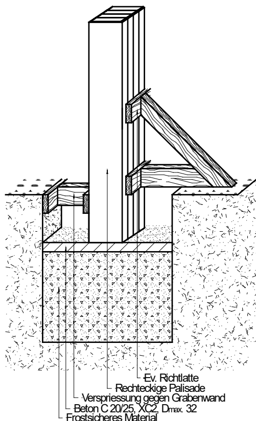
Bild 11: Einbau Palisaden
