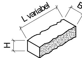
Bild 10: Technische Zeichnung SANTURO® Spaltmauerstein 2-seitig gespalten
