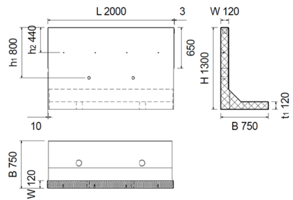
Bild 2: Perronwinkel Typ 2 (Standardtyp für Normalspurbahn)
