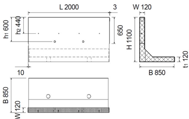
Bild 3: Perronwinkel Typ 3 (Standardtyp für Schmalspurbahn)
