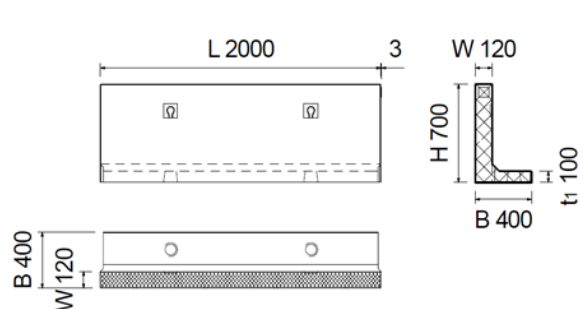
Bild 6: Perronwinkel Typ 6
