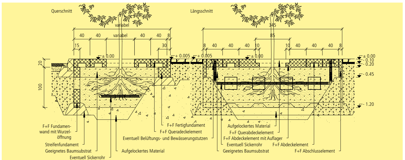
Einbauschema F+F Baumwurzelraumschutz mit Fundamentwand mit Wurzelöffnungen, Fertigteilfundament und Abschlusslement
