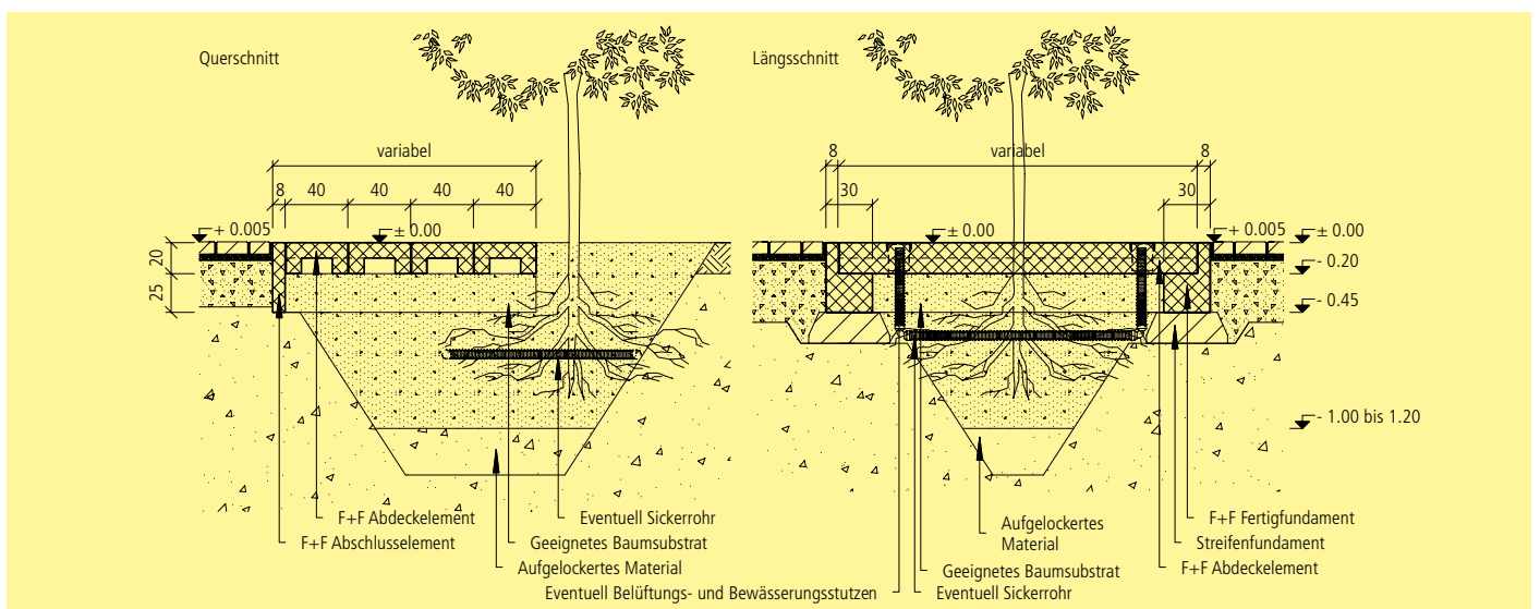
Einbauschema F+F Baumwurzelraumschutz als Wegbrücke mit Fertigteilfundament und einem Abschlusslement
