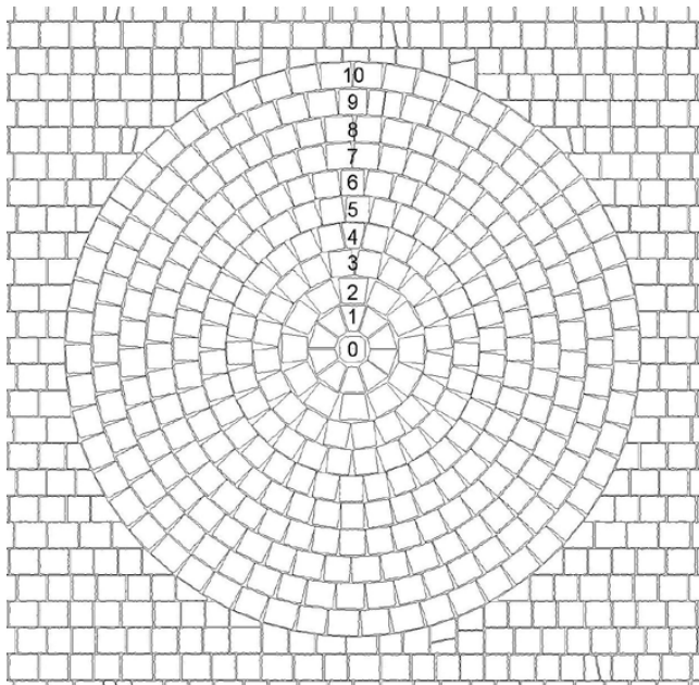
Kreisplasterung mit FRIEDA® Pflastersteinen
