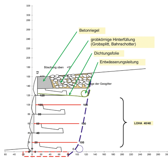
Diagramm 1: Dichtungsfolie und Entwässerungsleitung unterhalb des Grobsplittes oder Bahnschotter
