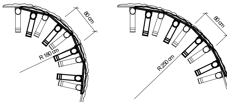
Bild 36: Kleine Radien z. B. R = 180 cm oder R = 250 cm
