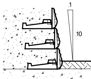
Bild 27: Wandneigung 1:10 (84°), Standard
