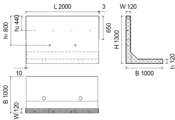
Bild 1: Perronwinkel Typ 1 (Standardtyp für Normalspurbahn)
