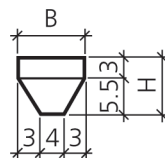
Bild 6: Abschlussbalken oben
