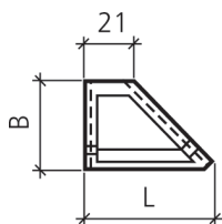
Bild 8: ECKELEM. Aussenecke links (ausspringend)
