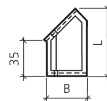
Bild 11: ECKELEM. Innenecke rechts (einspringend)
