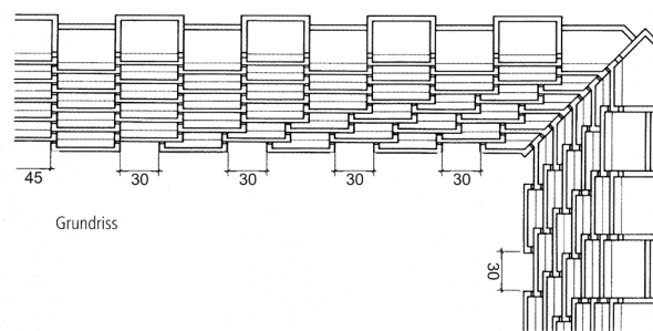
Bild 22: Grundriss Innenecke
