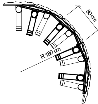
Bild 36: Kleine Radien z. B. R = 180\text{ cm} oder R = 250\text{ cm}
