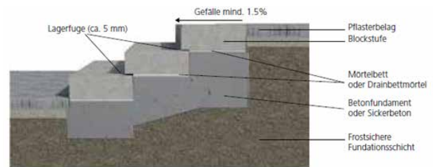
Bei der Blockstufe FROSTA LEGER muss das Fundament zwingend bis zur Aussenkante gezogen werden
